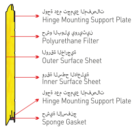
ع ب ص ا ل ا ق ص ر ق ق و ل ل ك ي ه Finger protection Panel Structure
