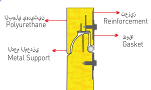
ف ي و و ر ك ي م ق و ل Microwave Panel
